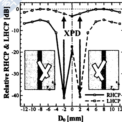
(b) RHCP & LHCP
